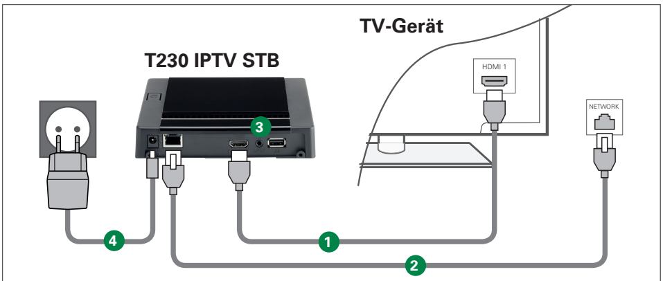
Abbildung 2 - Anschlussreihenfolge
