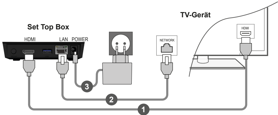
Abbildung 3: Kabelverbindungen
