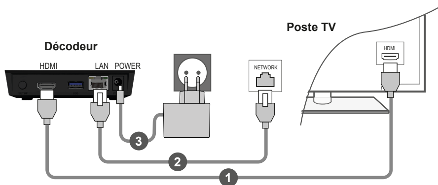
Figure 3 : Connexions par câbles
