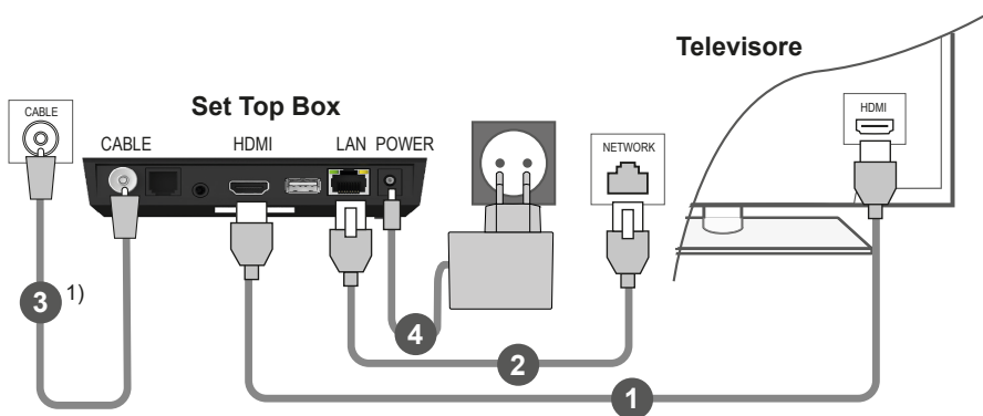
Figura 3: Collegamenti via cavo
