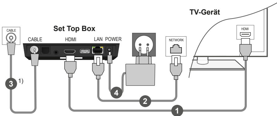
Abbildung 3: Kabelverbindungen
