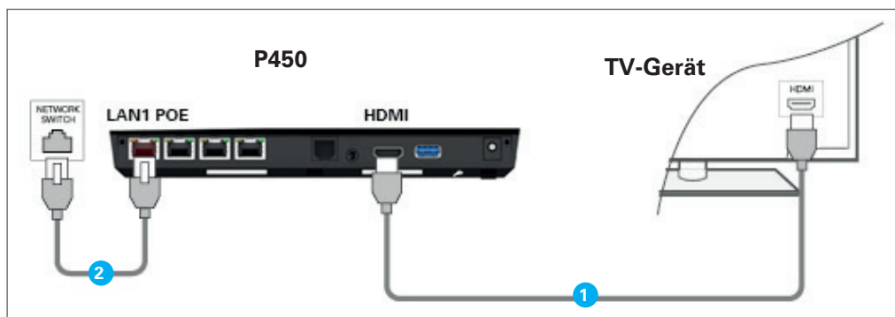
Abbildung 2 - Kabelverbindungen - PoE
