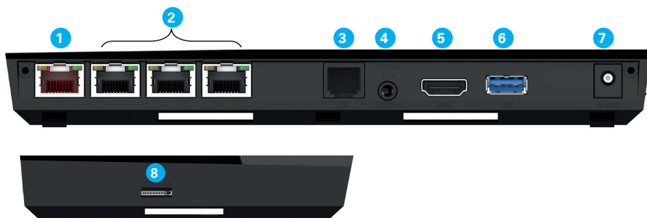
Abbildung 1 - Anschlüsse
