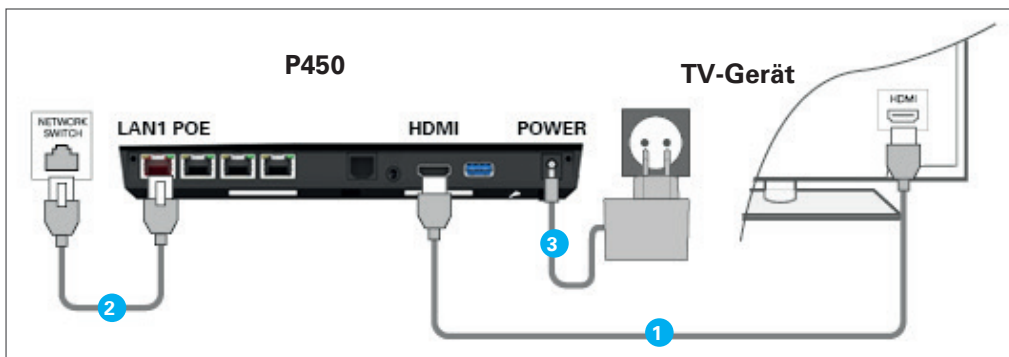
Abbildung 3 - Kabelverbindungen - Steckernetzteil
